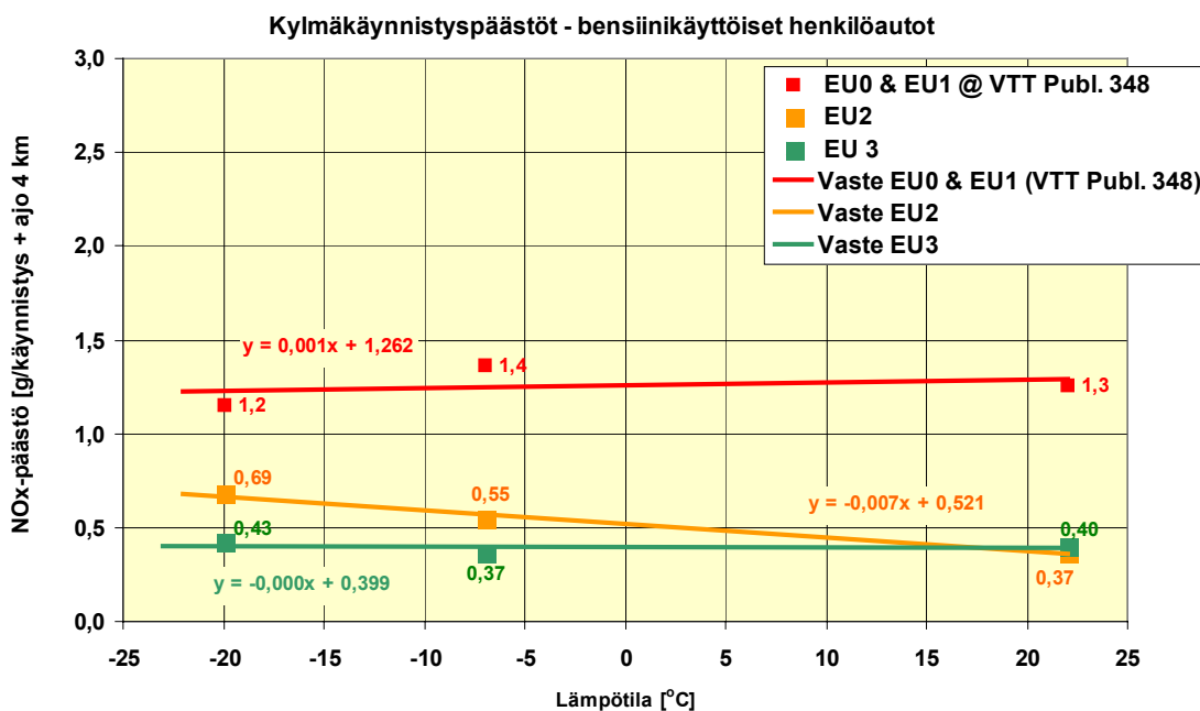
Kuva 1.12 Kylmäkäynnistyspäästöjen NOx-lisäpäästö käynnistyslämpötilan funktiona; bensiinikäyttöiset autot EU0 ... EU3.
