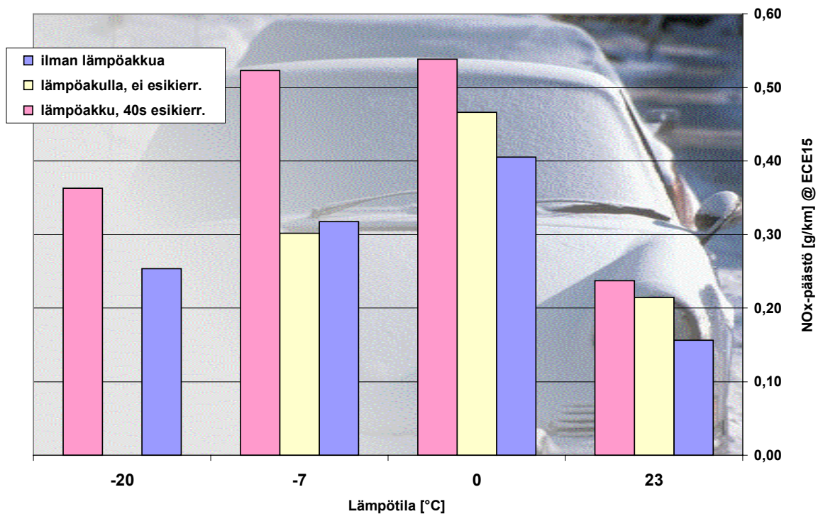
Kuva 2.6. NO x -päästöt eri koelämpötiloissa ilman lämpöakkaa ja akkua käytettäessä.
