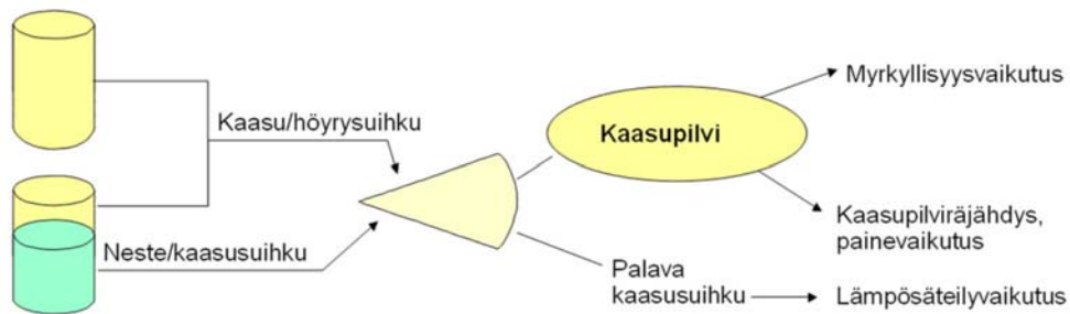
Kuva 4. Paineistetun säiliön vuodon yhteydessä syntyvät kaasuvuodot ja kaasujen erilaiset leviämismahdollisuudet.
