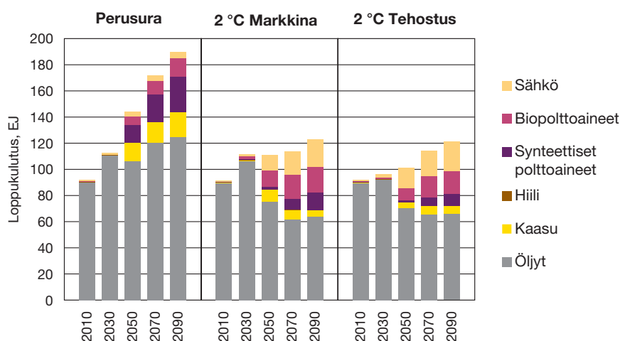
KUVA 8. Energian loppukäyttö liikennesektorilla Energy Visions 2050 -kirjan skenaarioissa. Sähköautot alkavat vallata markkinoita pienemmissä teholuokissa pyrittäessä rajoittamaan maapallon lämpeneminen kahteen asteeseen.
