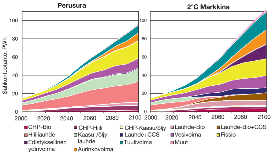
KUVA 19. Maailman sähköntuotanto pääluokittain Perusura- ja 2 °C Markkina -hillintäskenaariossa, jossa energianhankinnan rakenne optimoidaan 2 °C:n tavoitteen saavuttamiseksi. Kuvia vertailemalla näkyy selvä ero ilmastonmuutoksen hillinnän vaikutuksesta sähköntuotannon rakenteeseen. Laaja joukko eri teknologiovaihtoehtoja tarvitaan ilmastonmuutoksen hillitsemiseksi.
