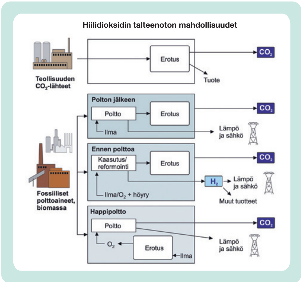
KUVA 10. Hiilidioksidin talteenoton mahdollisuudet. CO 2 :n erottamiseksi on kolme talteenottoteknologioiden pääluokkaa: erotus polton jälkeen, erotus ennen polttoa ja happipolttto, joiden välinen valinta riippuu mm. siitä, minkälaiseen voimalaitokseen CO 2 :n erotusta sovelletaan. Erotettu hiilidioksidi puuristetaan kokoon ja kuljetetaan varastointipaikalle putkessa tai laivalla. Soveltuvia varastointipaikkoja voivat olla mm. käytetyt öljy- ja kaasukentät ja muut soveltuvat geologiset muodostumat kuten suolakerrostumat. (Alkuperäinen kuva: IPCC 2005)
