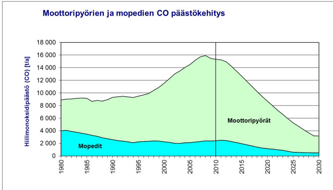
Kuva 17. Päästömallin laskema moottoripyörien ja mopediin hiilimonoksidipäästö.
