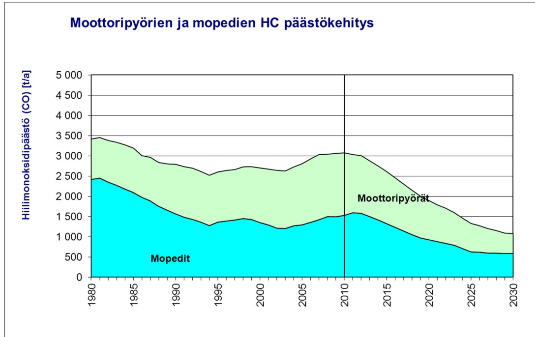
Kuva 19. Päästömallilla laskettu moottoripyörien ja mopeditien hiilivetyypäästöjen kehitys.
