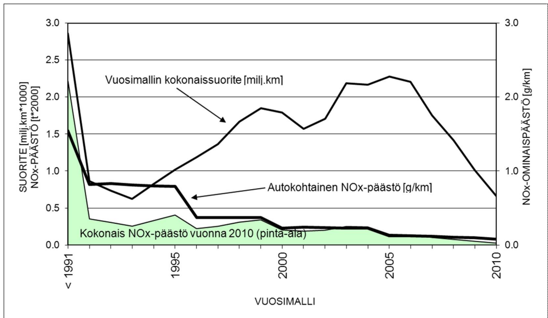
Kuva 21. Bensinikäyttöisten henkilöautojen vuosimallikohtaiset typenoksidipäästöt (NOx- päästöt) ja suoriteosuudet vuonna 2010. Vuoden 2010 mallit eivät ole olleet koko vuotta käytössä ja päästöt ovat siksi vain puolet vuoden lopun tilanteesta.
