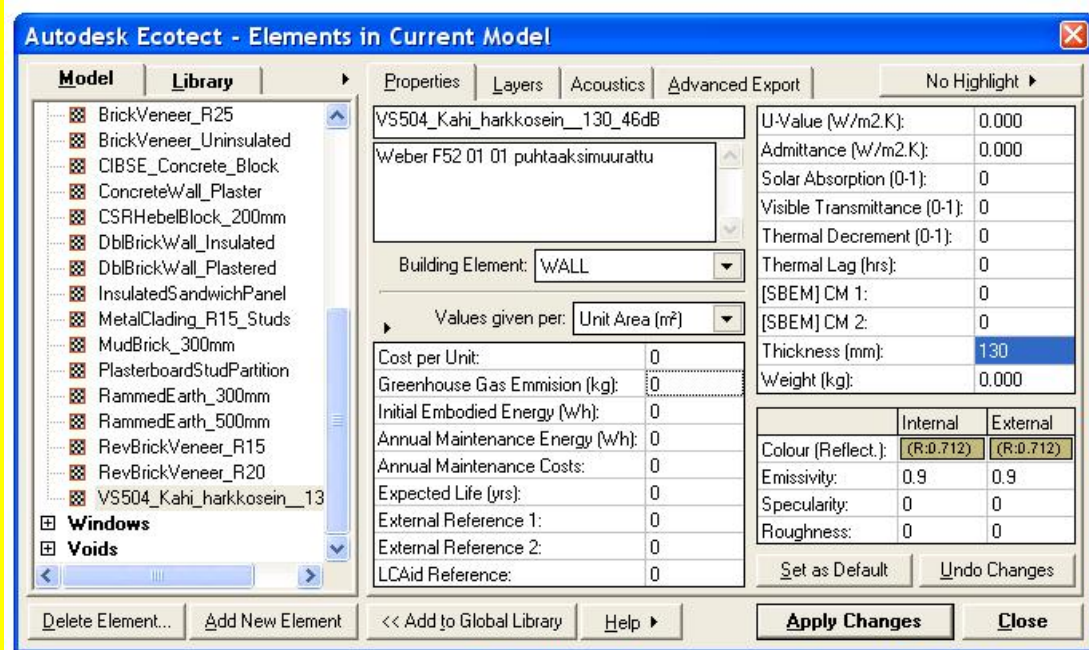
Kuva 16. Rakennetyypin ominaisuudet.
