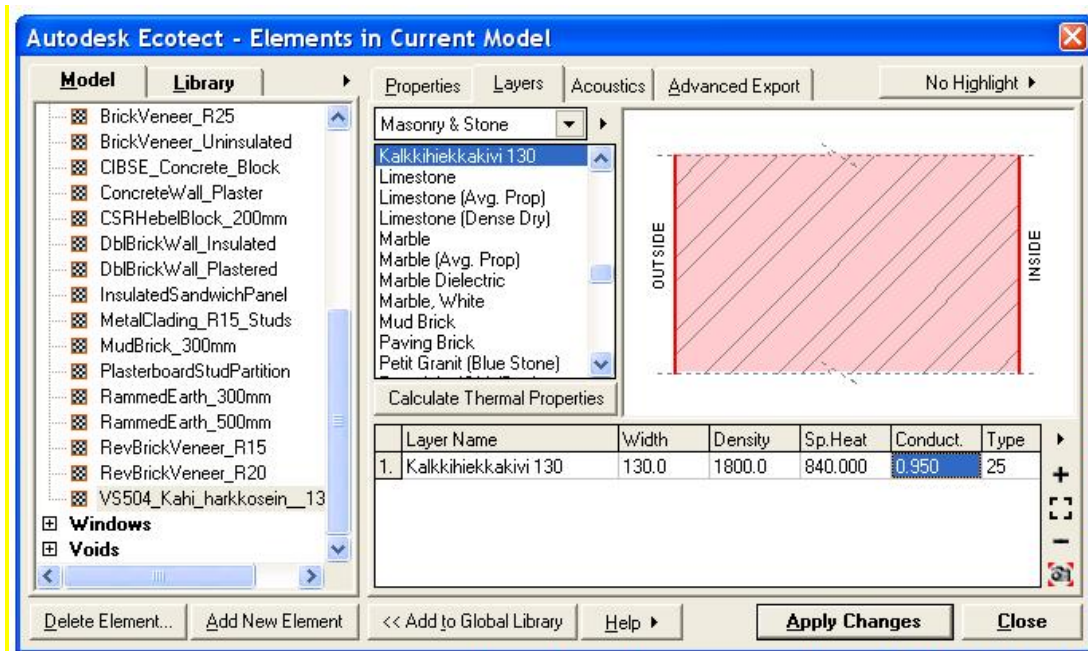
Kuva 17. Rakennekerroksen materiaaliominaisuudet.
