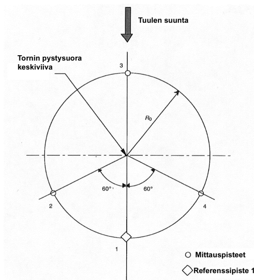
Kuva 2. Mittauspisteet standardin IEC 61400-11 mukaisesti [3].
