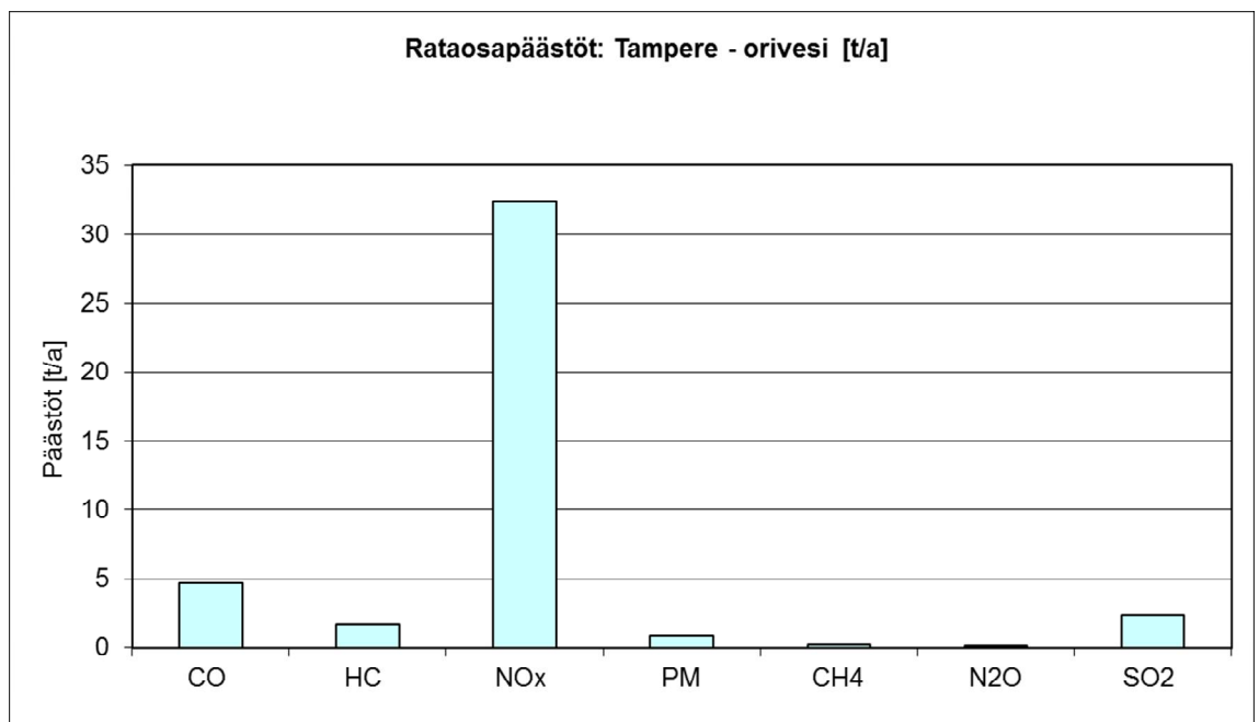
Kuva 6. Rataosan Tampere-Orivesi junaliikenteen päästöt 2012.
