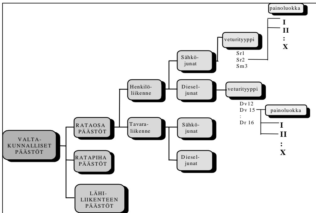
Kuva 1. Laskentamallin rakenne.
