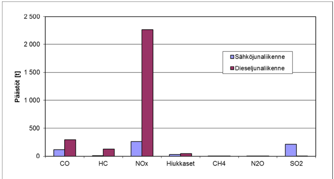
Kuva 5. Valtakunnalliset junaliikenteen päästöt 2012.
