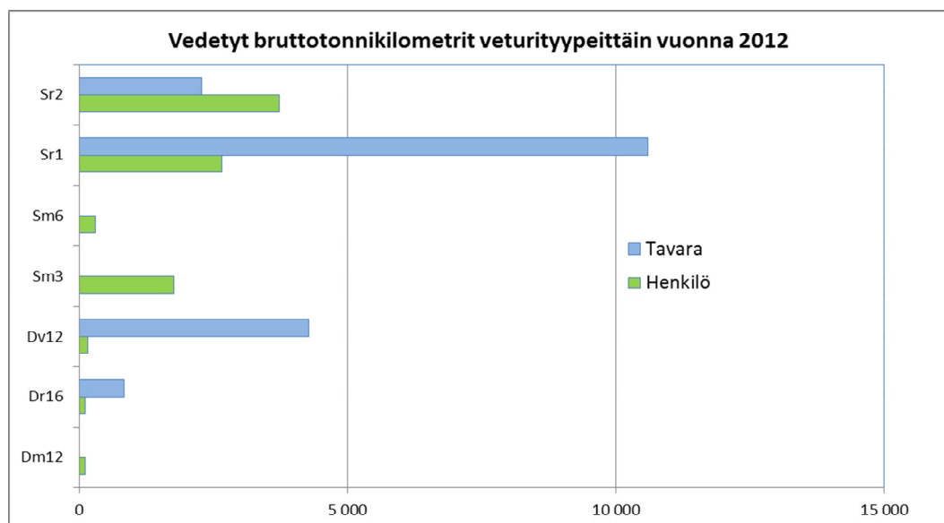
Kuva 3. Vedetyt bruttotonnikilometrit veturityypeittäin 2012.
