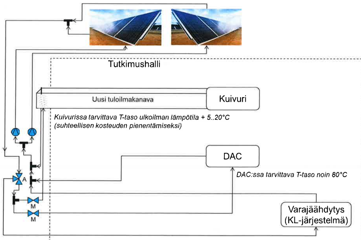
Kuva 16. Aurinkojärjestelmän periaatekuva
