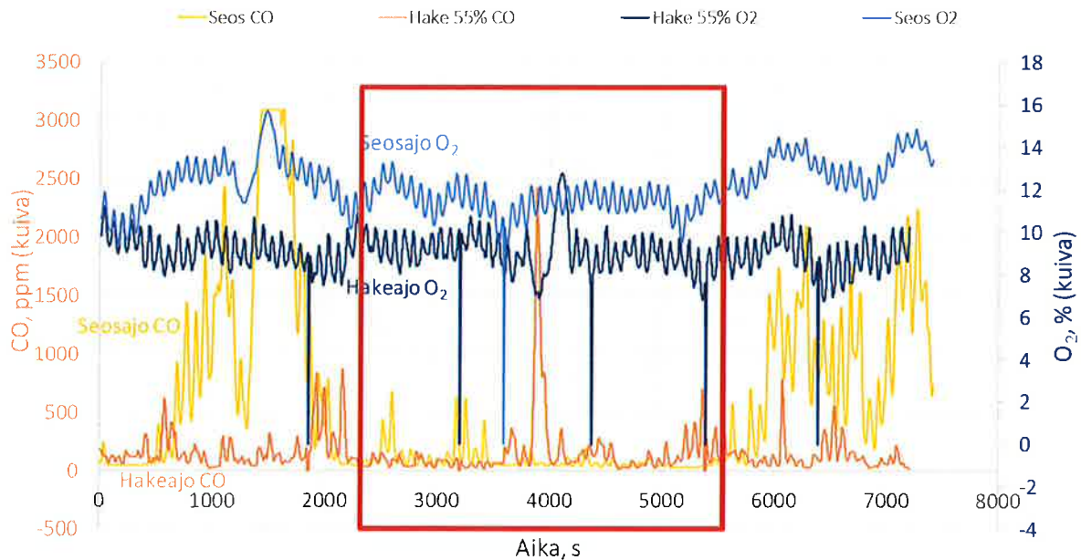
Kuva 9. Pellettien seostamisen vaikutus häkäpäästöihin hakkeen kosteudella 55 % nimellisteholla ajettaessa (~350 kW). Keskiarvot seospolttokokeen osalta on laskettu punaisella merkatus jakson ajalta, jolloin prosessi oli tasainen.
