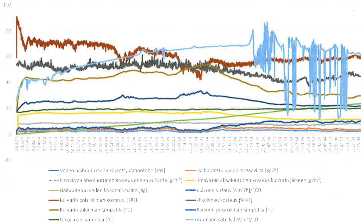
Kuva 18. Tuoreen rankahakkeen kuivauksen mittaustulokset 15.8.2017 kuivauskokeessa algoritmilla 2.
