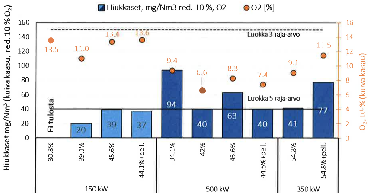
Kuva 11. Gravimetrisellä menetelmällä määritetyt keskimääräiset hiukkaspitoisuudet kuivassa kaasussa ( \text{mg}/\text{Nm}^3 ) ja redusoituna 10 %:n jäännöshappipitoisuuteen sekä mitattu jäännöshappi kuivassa kaasussa.
