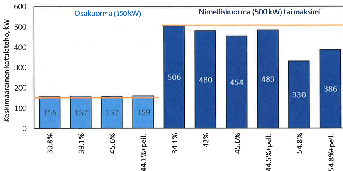
Kuva 4. Toteutuneet ja tavoitellut keskimääräiset kattilatehot.
