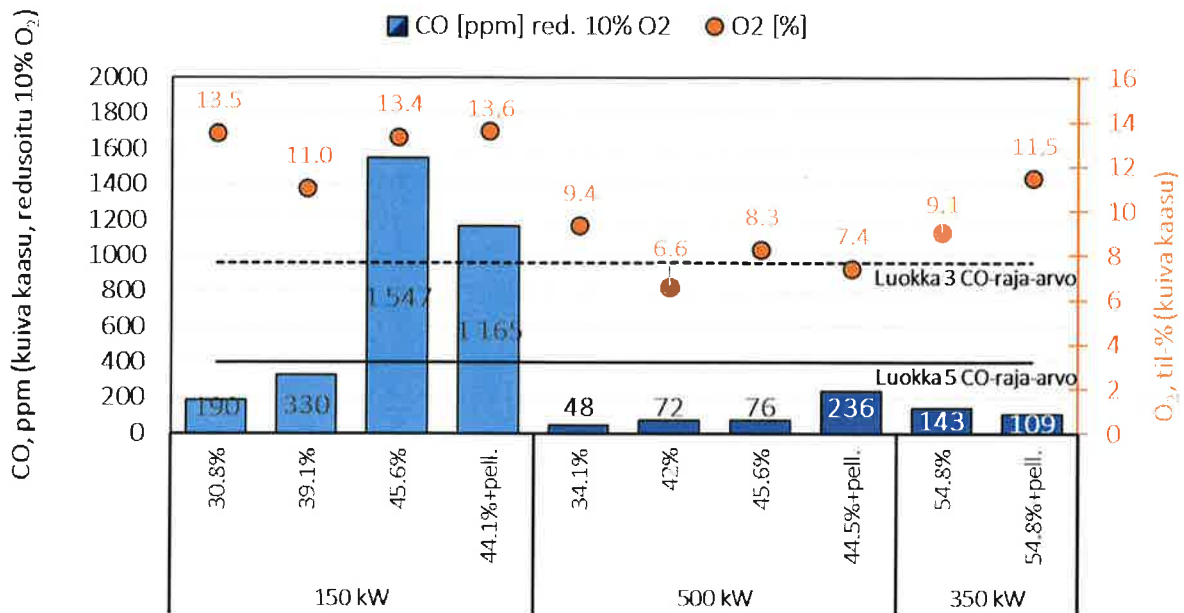
Kuva 6. Keskimääräiset häkäpäästöt kuivassa kaasussa ja redusoituna 10 %:n jäännöshappipitoisuuteen sekä mitattu jäännöshappi kuivassa kaasussa. (Muuntokerroin ppm → mg/Nm 3 = 1,25)
