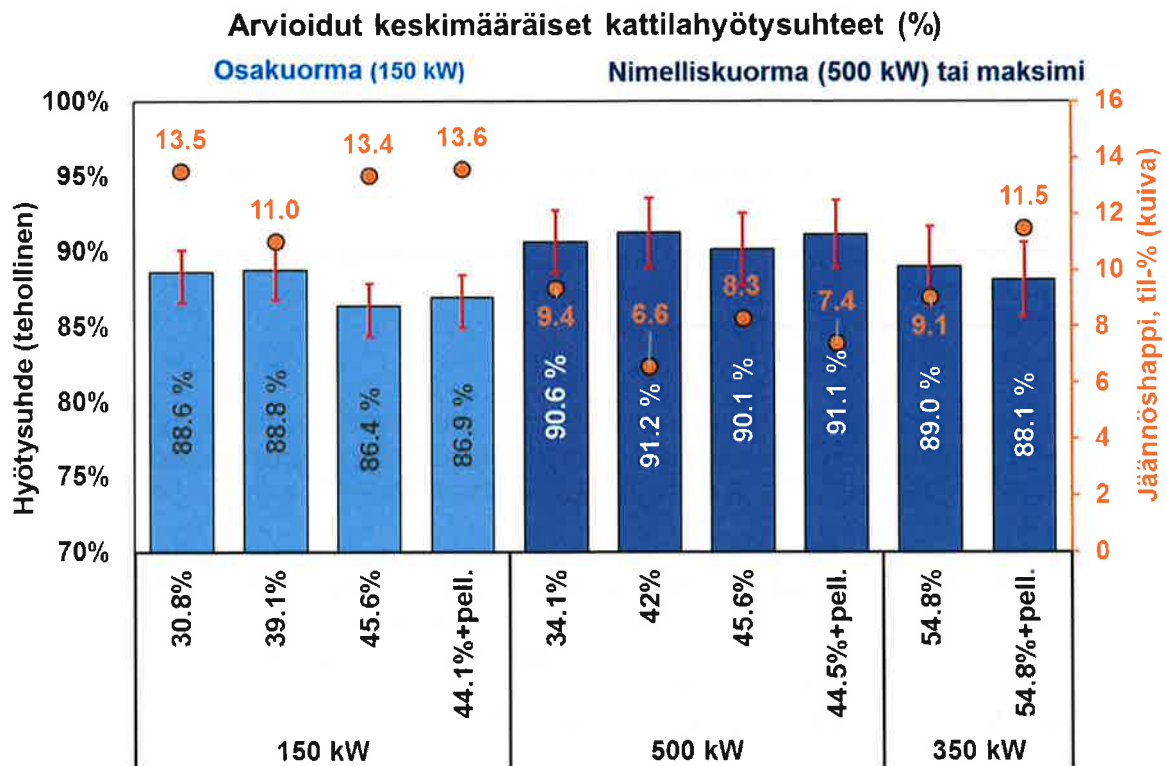
Kuva 5. Epäsuoralla menetelmällä laskennallisesti määritetyt keskimääräiset kattilahyötysuhteet.
