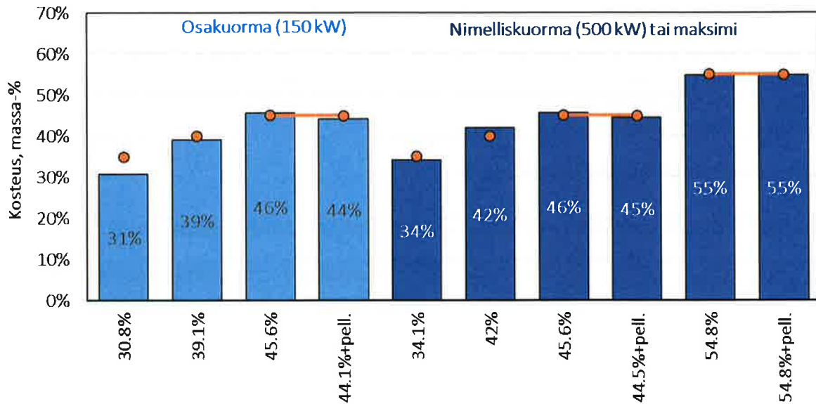
Kuva 3. Toteutuneet (sininen) ja tavoitekosteudet (oranssi) hakkeelle.
