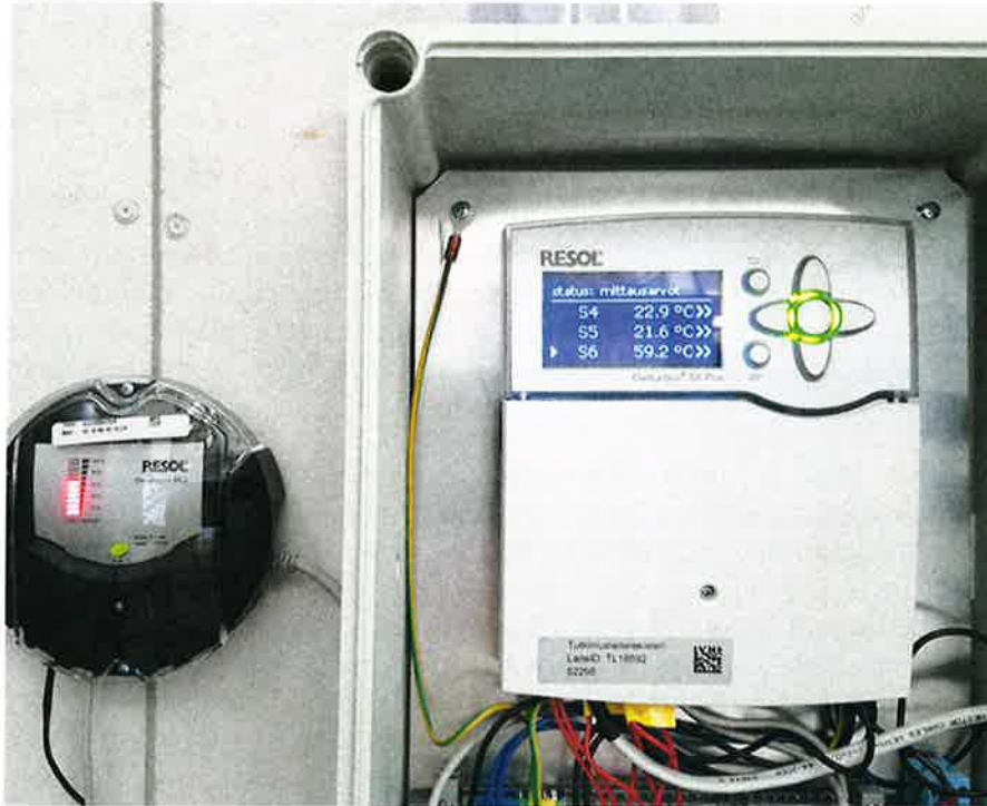
Kuva 15. Resol DeltaSol MX ohjausyksikkö.
