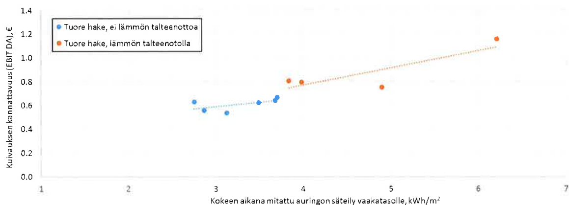
Kuva 20. Käyttökate tuoreen hakkeen kuivauksessa ennen ja jälkeen lämmön talteenoton. Hankkeen aikana asennetun lämmön talteenoton hyöty näkyy sekä soviteen tasokorotuksena että jyrkempänä kulmakertoimena johtaen merkittävään eroon vuositason kannattavuudessa.
