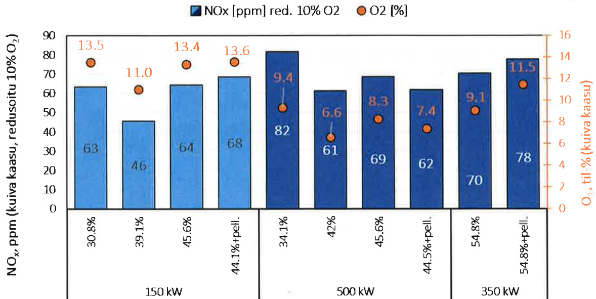
Kuva 10. Keskimääräiset typenoksidipäästöt kuivassa kaasussa ja redusoituna 10%:n jäännöshappipitoisuuteen sekä mitattu jäännöshappi kuivassa kaasussa. (Muuntokerroin ppm \rightarrow mg/Nm 3 NO 2 = 2,05)
