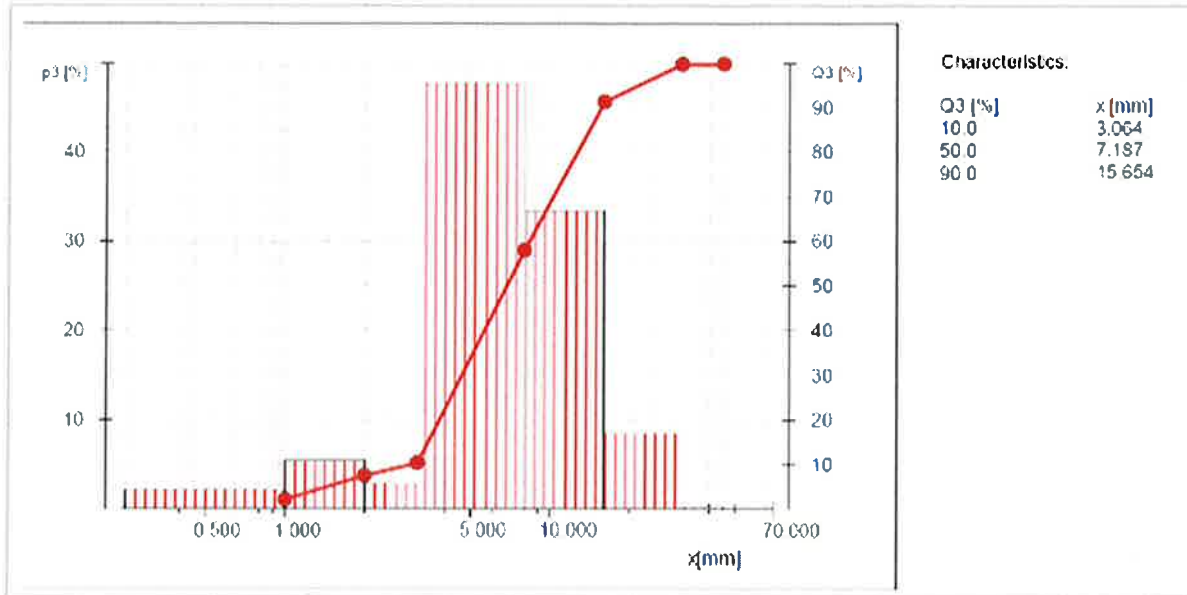
Kuva 17. Hakkeiden palakokojakauma.
