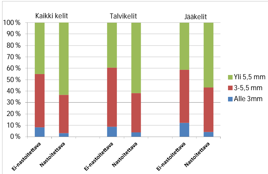
Kuva 6. Onnettomuuden A-osallisten huonoimman renkaan urasyvyys talvirenkaan tyypin ja kelin mukaan. Tarkastelussa mukana vain henkilö- ja pakettiautojen talvirenkaat kuolemaan johtaneissa onnettomuuksissa vuosina 1997–2012. Kesä- tai sekarenkain aiheutetut onnettomuudet sekä itsemurhat, nukahtamiset ja sairauskohtaukset on rajattu tarkastelun ulkopuolelle.
