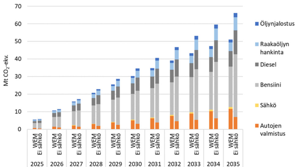
Kuva 50. Henkilöautojen sähköistymisen vaikutus kumulatiivisiin kasvihuone-kaasupäästöihin vuosina 2025–2035 WEM-skenaariossa. "Ei sähkö" -skenaariossa kaikki uudet henkilöautot ovat polttomoottorikäyttöisiä.
