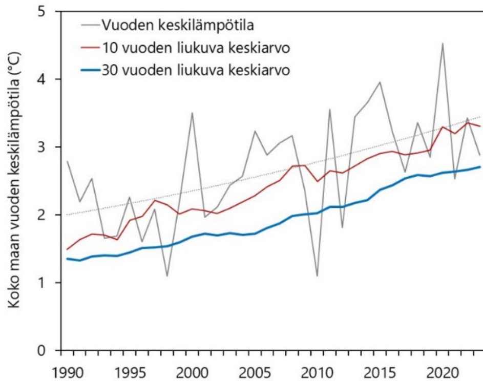
Kuva C5. Koko Suomen vuoden keskilämpötila ja sen 10 ja 30 vuoden liukuva keskiarvo. Harmaa katkoviiva on keskilämpötilojen lineaarinen trendi vuosille 1990–2023.
