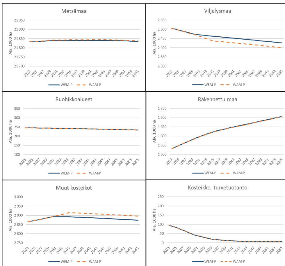
Kuva 8. Maankäyttöluokkien pinta-alojen kehitys vuosina 2023–2055 WEM- ja WAM-skenaarioissa.
