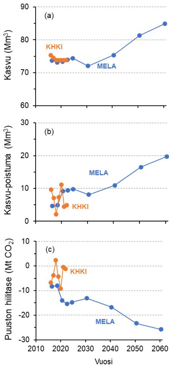
Kuva C2. MELA-ohjelmiston tuottama ja kasvihuonekaasuinventaarion (KHKI) vuosille 2016–2022 raportoima Etelä-Suomen puuston (a) runkotilavuuden kasvu, (b) runkotilavuuden kasvun ja poistuman erotus, ja (c) hiilitase. Vuosille 2016–2022 MELA-skenaariossa käytettiin rajoitteena kyseisten vuosien tilastoituja hakkuukertymiä. Skenaario toteutettiin kahden vuoden laskentakausina (skenaariota jatkettiin 10 vuoden laskentakausilla ja viimeisen kaksivuotiskauden hakkuurajoitteella vuoteen 2060 asti). MELA-skenaariossa hiilitase laskettiin laskentakausien välisistä biomassavaraston muutoksista.
