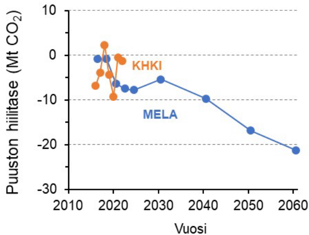
Kuva C4. MELA-ohjelmiston tuottama ja kasvihuonekaasuinventaarion (KHKI) vuosille 2016–2022 raportoima Etelä-Suomen puuston hiilitase, kun MELA-skenaariossakin runkopuun kasvu ja poistuma muunnettiin biomassaksi inventaarion käyttämällä muuntokertoimilla ja hiilitase laskettiin biomassakasvun ja -poistuman erotuksena.
