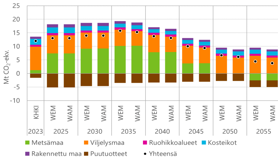
Kuva 29. Maankäyttösektorin päästö- ja poistumakehitys maankäyttöluokittain WEM- ja WAM-skenaariossa. Positiivinen luku on päästö ja negatiivinen poistuma (nielu). Vuosi 2023 vastaa KHK-inventaarion arvoja (Tilastokeskus 2025a).
