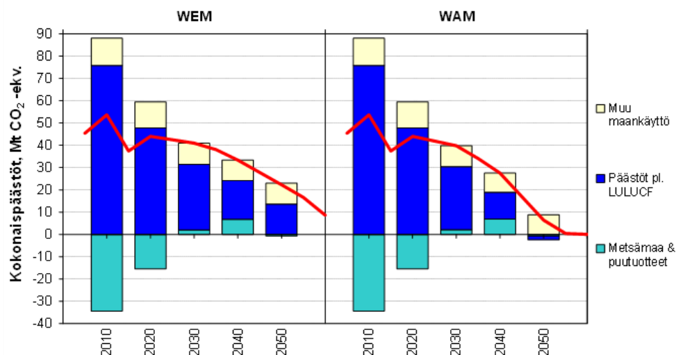
Kuva 31. Kasvihuonekaasupäästöjen ja -poistumien kokonaistase WEM- ja WAM-skenaariossa 2010–2050.
