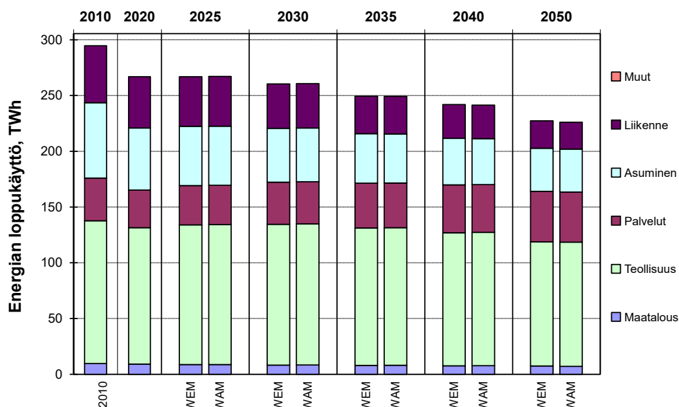
Kuva 18. Energian loppukulutus sektoreittain WEM- ja WAM-skenaariossa vuoteen 2050.
