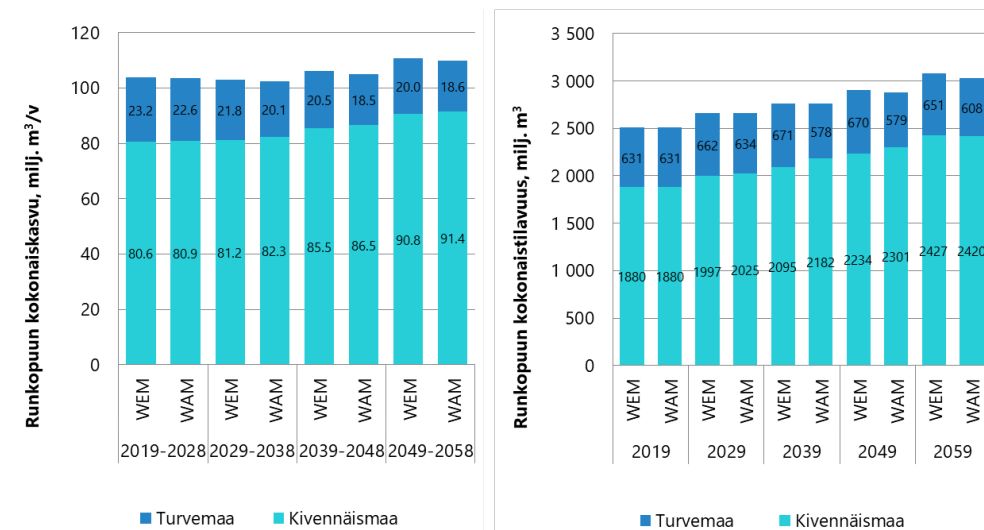
Kuva 12. Runkopuun a) vuotuinen kokonaiskasvu ja b) kokonaistilavuus 10-vuotiskausittain koko metsä- ja kitumaalla WEM- ja WAM-skenaarioiden mukaan koko maassa.
