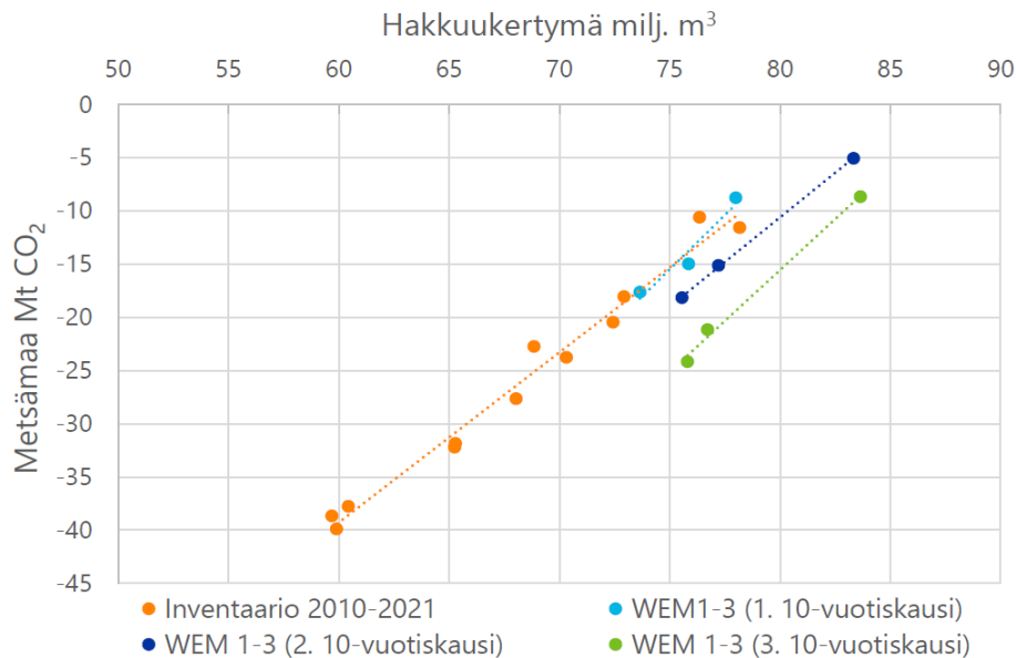
Kuva 7. Runkopuun hakkuukertymän (Mm 3 ) ja metsämaan CO 2 -nielun (Mt CO 2 ) suhde kasvihuonekaasuinventaarion tuloksissa (vuodet 2010–2021, oranssi) ja skenaariomallinnusten kolmella ensimmäisellä 10-vuotiskaudella (WEM1-3 ensimmäinen 10-vuotiskausi, vaaleansininen; WEM1-3 toinen 10-vuotiskausi, tummansininen; WEM1-3 kolmas 10-vuotiskausi, vihreä).
