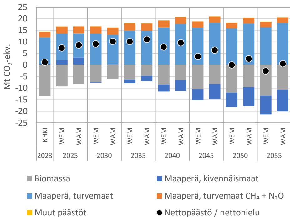
Kuva D1. Metsämaan kasviuonekaasupäästöjen ja -poistumien kehitys WEM- ja WAM-skenaariossa eriteltynä hiilivarastoihin ja päästölähteisiin, kun metsävarojen kehitysarvio on WAM-skenaarion mukainen. Positiivinen luku on päästö ja negatiivinen poistuma (nielu). Muut päästöt sisältävät typpilannoituksen, typen mineralisaation sekä maastopalojen, kulituksen ja ennallistamispolttojen päästöt. Vuosi 2023 vastaa KHK-inventaarion arvoja (Tilastokeskus 2025a).
