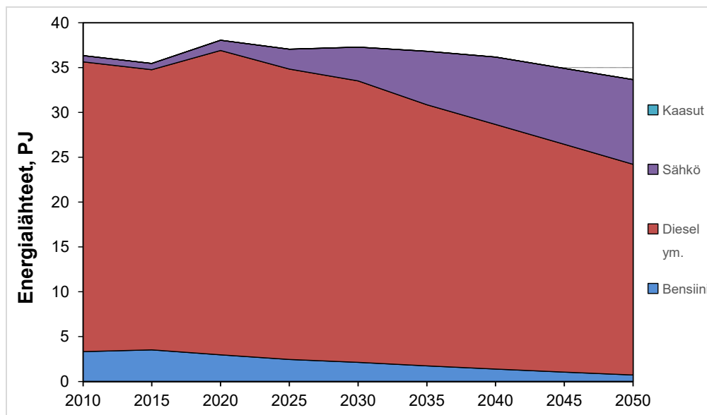
Kuva 23. Työkoneiden energialähteiden kehitys WEM-skenaariossa. WAM-skenaari- on kehitys poikkeaa tästä vain hieman suuremmin sähköistymisin.
