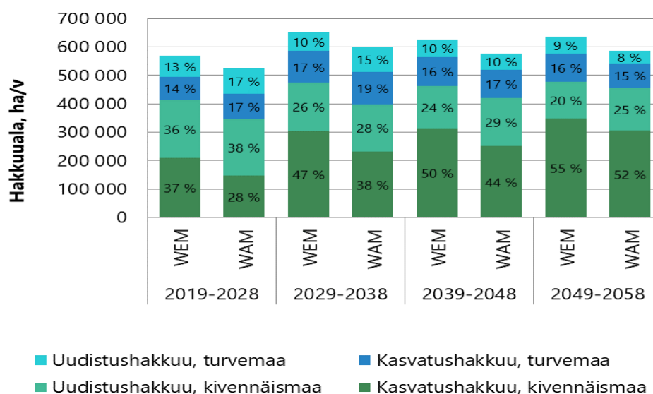
Kuva 10. Kasvatus- ja uudistushakkuiden vuotuiset pinta-alat puuntuotannossa olevalla metsämaalla WEM- ja WAM-skenaarioiden mukaan koko maassa 10-vuotiskausittain. Kasvatushakkuualaan sisältyvät harvennushakkuiden ja ylispuiden poistoon tähtäävien hakkuiden pinta-alat.
