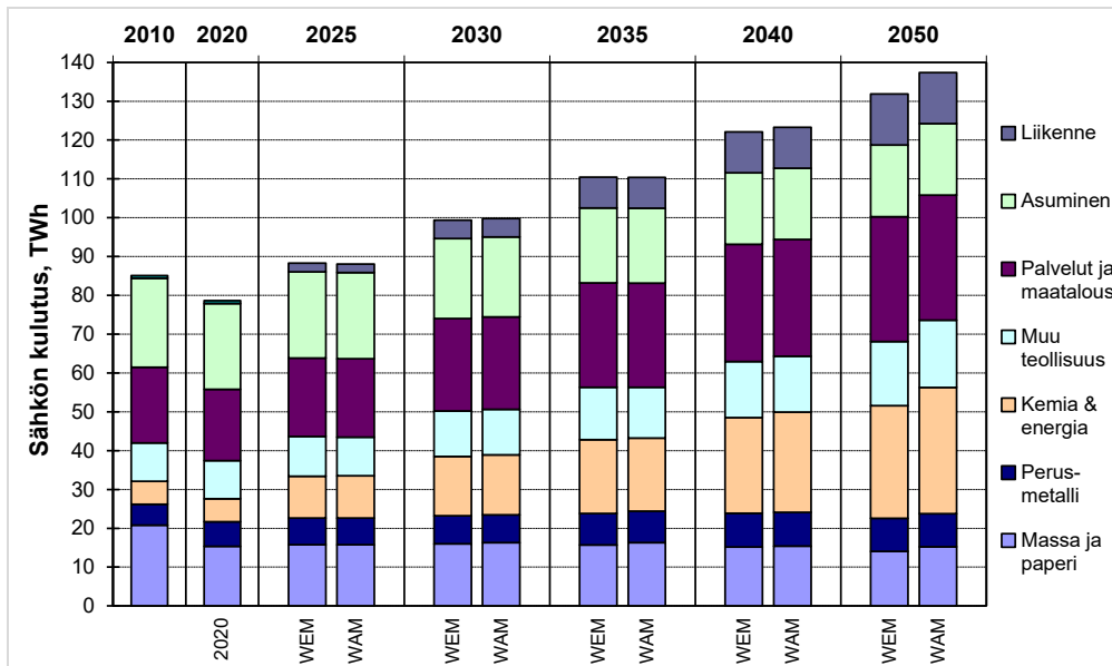
Kuva 19. Sähköenergian loppukulutus sektoreittain WEM- ja WAM-skenaariossa.
