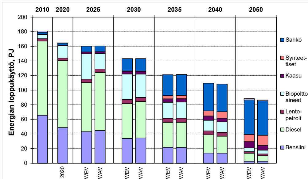
Kuva 21. Kotimaanliikenteen loppuenergian kulutus WEM- ja WAM-skenaariossa vuoteen 2050.
