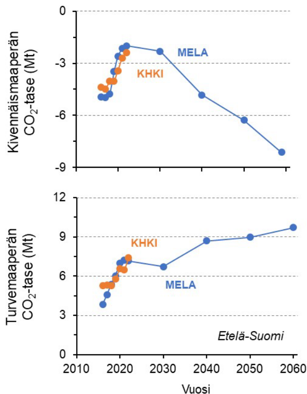
Kuva C3. MELA-ohjelmiston tuottama ja kasvihuonekaasuinventaarion (KHKI) raportoima Etelä-Suomen kivennäis- ja turvemaaperien CO 2 -tase vuosille 2016–2022. MELA-skenaariot yksityiskohdat kuten kuvassa C2.
