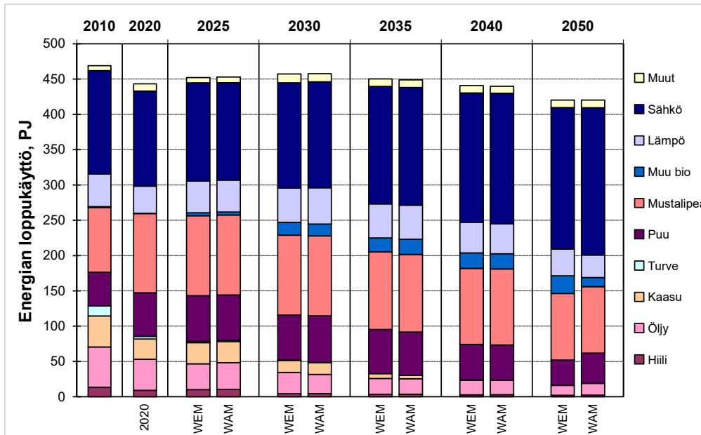
Kuva 22. Teollisuuden energian loppukulutus kulutus WEM- ja WAM-skenaariossa.
