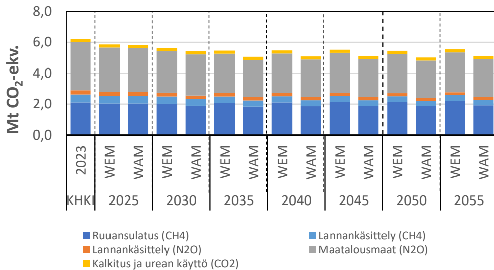
Kuva 7. Maatalouden päästöt WEM- ja WAM-skenaarioissa päästöluokittain. Vuosi 2023 vastaa KHK-inventaarion arvoja (Tilastokeskus 2025a).
