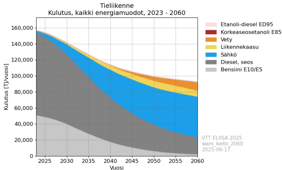
Kuva 4. Energiankulutuksen kehitys polttoaineittain tieliikenteen WAM-skenaariossa vuosina 2023–2060.
