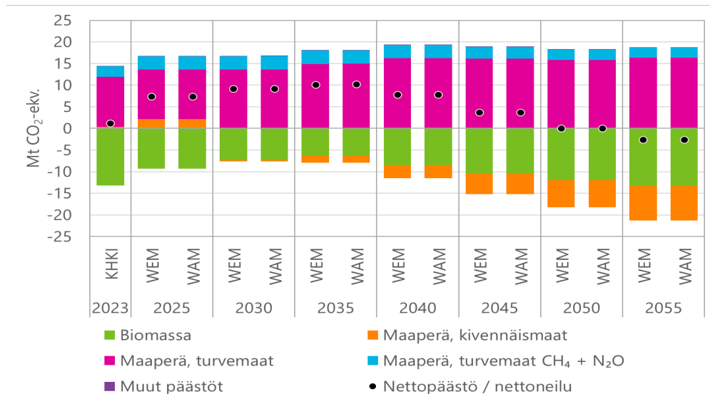
Kuva 30. Metsämaan kasvihuonekaasupäästöjen ja -poistumien kehitys WEM- ja WAM-skenaariossa eriteltynä hiilivarastoihin ja päästölähteisiin. Positiivinen luku on päästö ja negatiivinen poistuma (nielu). Muut päästöt sisältävät typpilannoituksen, typen mineralisaation sekä maastopalojen, kulutuksen ja ennallistamispolttojen päästöt. Vuosi 2023 vastaa KHK-inventaarion arvoja (Tilastokeskus 2025a).
