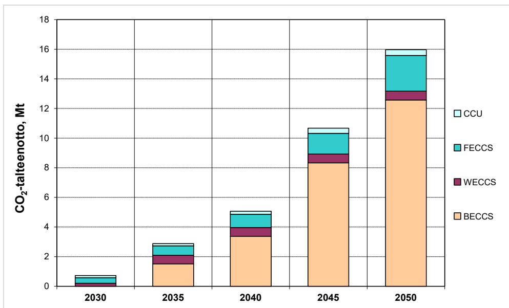
Kuva 26. Hiilidioksidin talteenoton kehitys WAM-skenaariossa 2030–2050.
